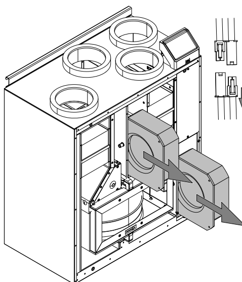
Fig. 6 Avtrekks- og tilluftvifter
