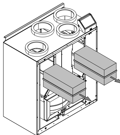
Fig. 4 Avtrekks- og tilluftfilter
