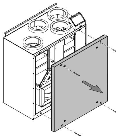
Fig. 3 Ta av og sette på det indre dekselet
